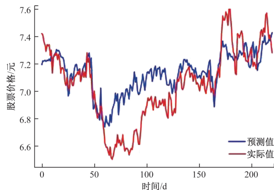
图6 ISOMAP-LSTM 模型预测曲线
