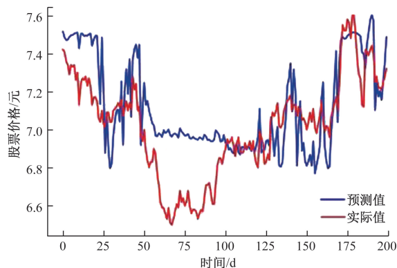
图4 MAH-LSTM 模型预测曲线
