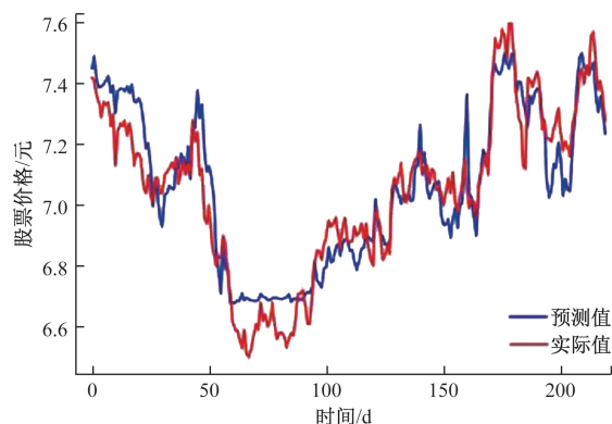
图5 PCA-LSTM 模型预测曲线图
