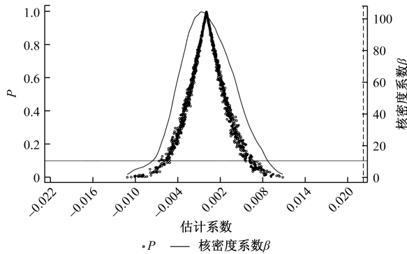
图2 安慰剂检验
