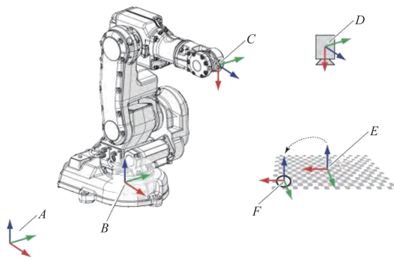
图2 相机与工业机器人手眼标定
